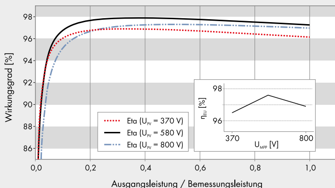
Wirkungsgradkurve SUNNY TRIPOWER 10000TL
